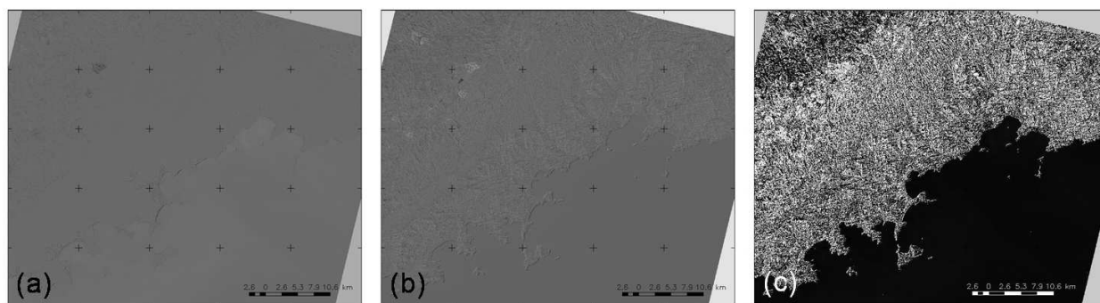
Figura 5. Imagem detecção de mudança. (a) imagem intermediária banda vermelho; (b) imagem intermediária banda infravermelho próximo; e (c) imagem detecção final. Tamanho do pixel: 30x30m.
