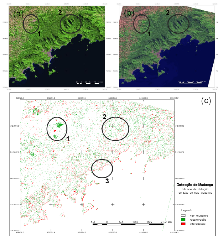
Figura 6. Imagens e mapa de detecção de mudança da área de estudo. (a) Imagem Landsat TM de 2004; (b) Imagem SPOT XS de 2006; e (c) Mapa de detecção de mudança entre 2004 e 2006, obtido a partir da técnica de rotação radiométrica por eixo de não mudança (RCEN).
